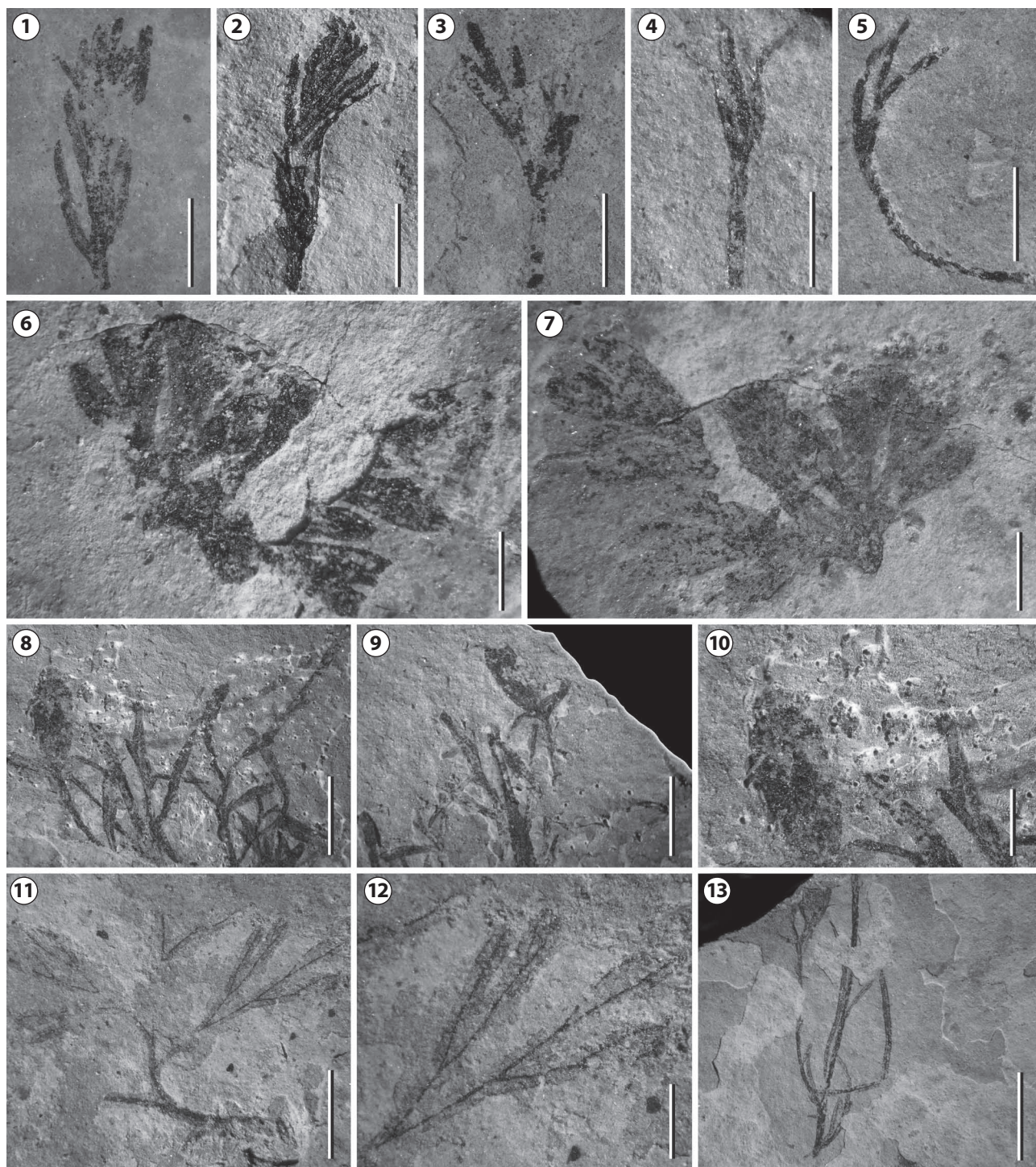
Figura 6. Macrofósiles de Briofitas/ Bryophytic macrofossils . 1-5 , Thallites sp. Fragmentos de talo, el eje se ramifica dicotómicamente y las ramificaciones son lineales/ fragments of thallus, axis branches dichotomously and linear branches ; 1 , (MHIN-UNSL-GEO-P611); 2 , (MHIN-UNSL-GEO-P612); 3 , (MHIN-UNSL-GEO-P613); 4 , (MHIN-UNSL-GEO-P614); 5 , (MHIN-UNSL-GEO-P615); 6-7 , cf. Hepaticites sp. 2, fragmento de talo, ramificaciones lobuladas que forman un abanico/ fragment of thallus, lobed, fan-like branches ; 6 , (MHIN-UNSL-GEO-P617 a) y 7 , (MHIN-UNSL-GEO-P617 b); 8-10 , Muscites sp., gametofito con numerosas hojas lineares o lanceoladas/ gametophyte with many linear or lanceolate leaves ; 8 y 10 , (MHIN-UNSL-GEO-P618 a); 9 , (MHIN-UNSL-GEO-P618 b); 8 , esporofito acrocárpico con cápsula erecta y peristoma formado por dientes/ acrocarpous sporophyte with erect capsule and peristome formed by teeth ; 9 , esporofito acrocárpico con cápsula erecta/ acrocarpous sporophyte with erect capsule ; 10 , detalle de cápsula/ detail of capsule ; 11-12 , cf. Hepaticites sp. 1 (MHIN-UNSL-GEO-P616), fragmento de planta postrada talosa/ fragment of prostrate plant thaloid ; 11 , ramificación dicotómica/ dichotomous branching ; 12 , detalle de la vena media en cada bifurcación/ detail of the midrib in each bifurcation ; 13 , “Fósil taloide indeterminado” (MHIN-UNSL-GEO-P619); fragmento de talo con hojas lanceoladas/ fragment of thallus with lanceolate leaves . Escala gráfica/ scale bar : para/ for 1, 10, 11 = 2,5mm; para/ for 8, 9, 13 = 5mm; para/ for 2 = 0,5 mm; para/ for 3, 5 = 2mm; para/ for 6, 7, 12 = 1mm; para/ for 4 = 1,5mm.
