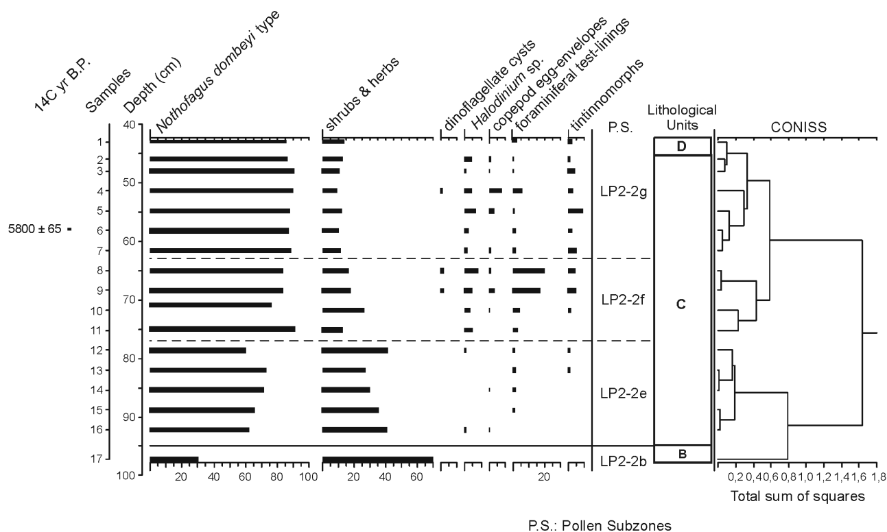
Figure 4. Palynomorph total frequency (%) at Bahía Lapataia 2 section / frecuencia total de polinórfos (%) en la sección de Bahía Lapataia 2.
