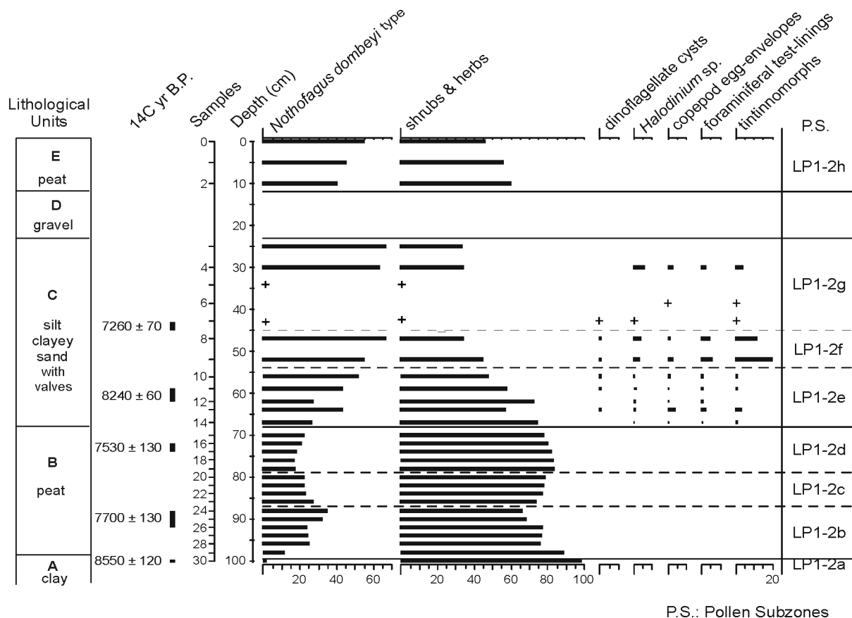
Figure 2. Palynomorph total frequency (%) at Bahía Lapataia 1 section (modified from Borrromei and Quattrocchio, 2001) / frecuencia total de palinórfos (%) en la sección de Bahía Lapataia 1 (modificado de Borrromei y Quattrocchio, 2001).
