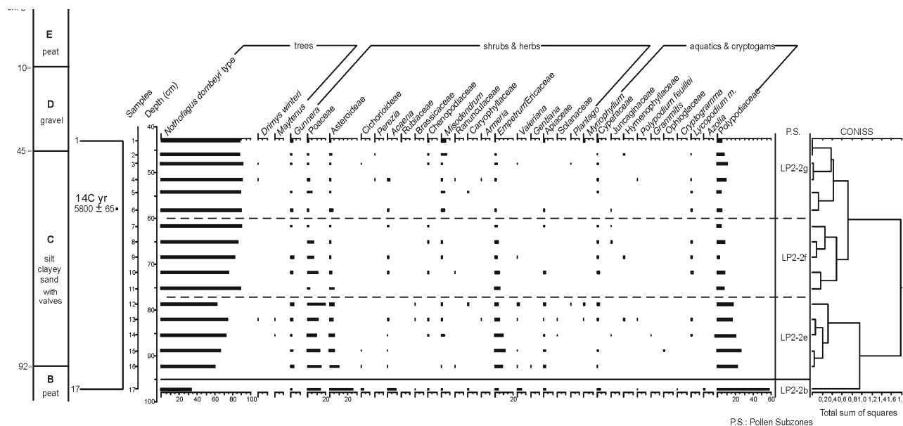
Figure 3. Pollen/spore frequency (%) at Bahía Lapataia 2 section / frecuencia de polen/esporas (%) en la sección de Bahía Lapataia 2.
