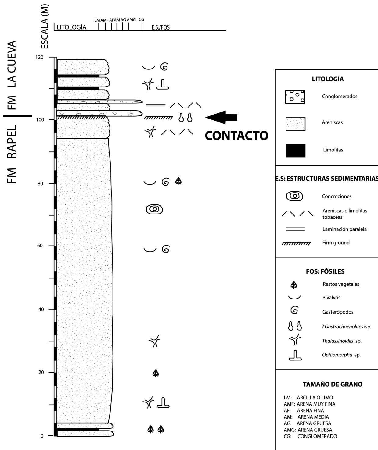
Figura 2. Sección estratigráfica de Cuesta de Los Leones (véase ubicación en figura 1). La discontinuidad entre las Formaciones Navidad (Miembro Rapel) y La Cueva está indicada por una flecha / stratigraphic section of Cuesta de Los Leones (see location in figure 1). Discontinuity between the Navidad (Rapel Member) and La Cueva Formations indicated by an arrow.
