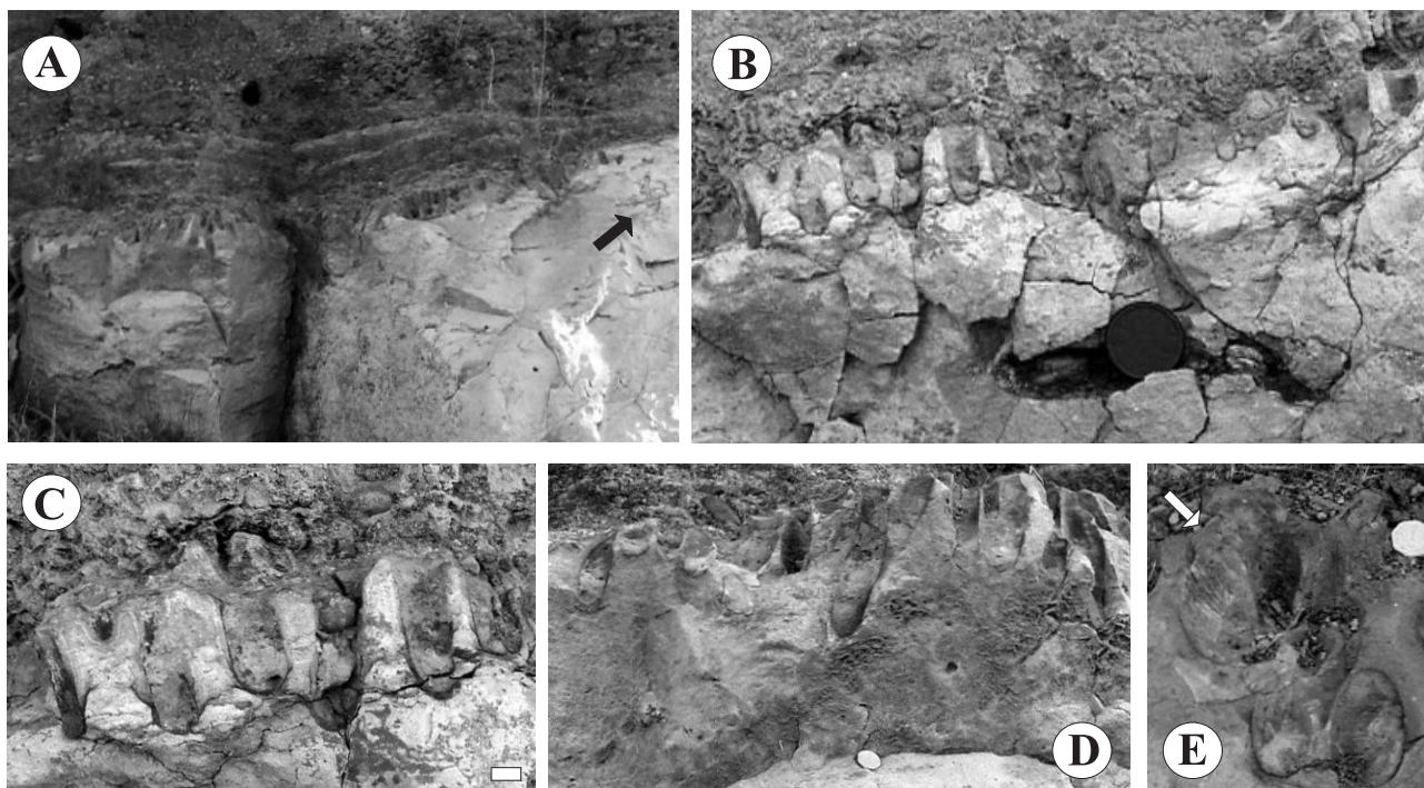
Figura 3. Icnofauna en el contacto entre las formaciones Navidad (Miembro Rapel) y La Cueva / Ichnofauna at the contact between the Navidad (Rapel Member) and La Cueva formations. A, Vista general del contacto entre ambas unidades caracterizado por abundantes ejemplares de ?Gastrochaenolites isp. y escasos Thalassinoides isp. (flecha) / general view of the contact between both units characterized by abundant ?Gastrochaenolites isp. and scarce Thalassinoides isp. B, Detalle de la superficie mostrando alta densidad de ?Gastrochaenolites isp. / close up of the surface showing high density of ?Gastrochaenolites isp. C, ?Gastrochaenolites isp. mostrando morfologías cilíndricas y, más raramente, en forma de gota / ?Gastrochaenolites isp. displaying cylindrical to, more rarely, drop-shaped morphology. D, Ejemplos de ?Gastrochaenolites isp. elongados y relativamente profundos / examples of elongate, relatively deep ?Gastrochaenolites isp. E, Detalle mostrando un molde interno de bivalvo preservado (flecha) / close-up showing bivalve internal mold preserved (arrow). Cubre del lente, 5.5 cm; Barra de escala, 1 cm; Moneda, 1,6 cm / lens cap is 5.5 cm; Scale bar is 1 cm; Coin is 1.6 cm.
