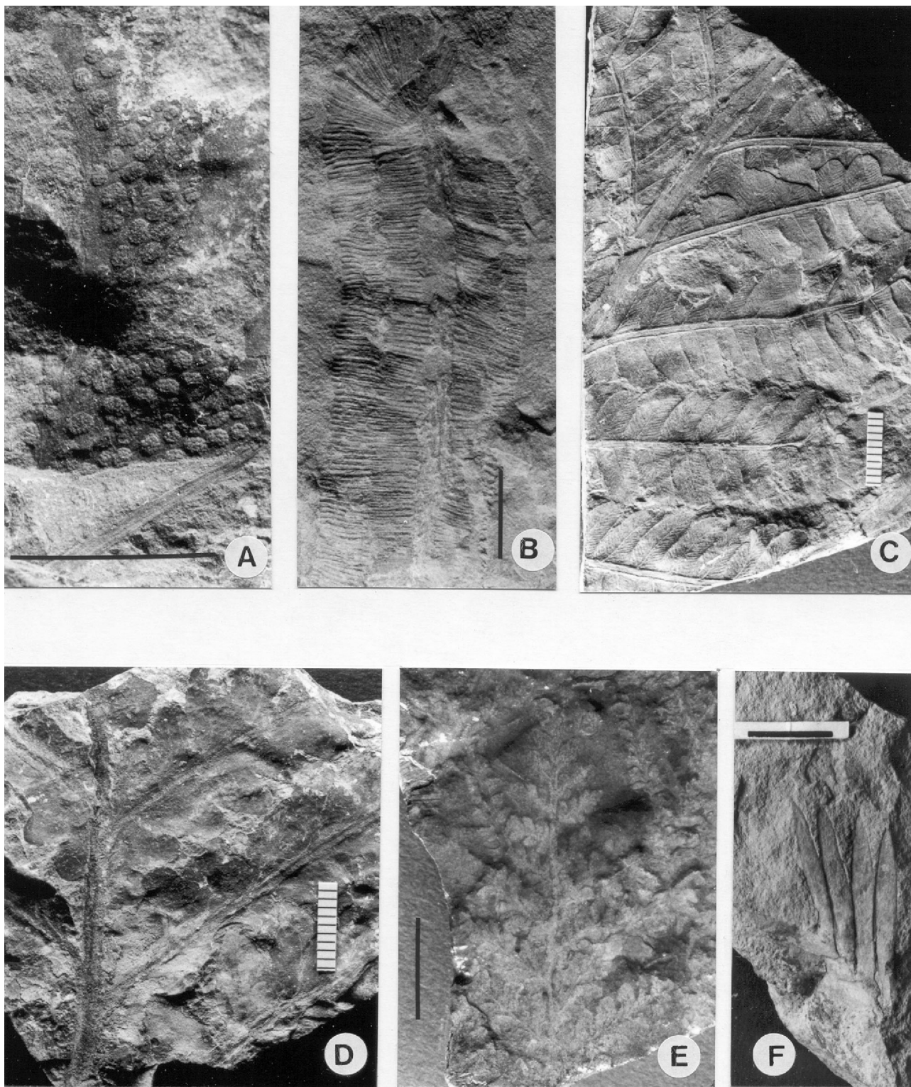
Figura 4. A, cf. Rienitsia colliveri Herbst LPPB 13173; B, Marattia münsteri (Goeppert) Zeiller LPPB 14174; C, Cladophlebis oblonga LPPB 13182; D, Archangelskya proto-loxsoma (Kurtz) Herbst LPPB 13200; E, Scleropteris vincei Herbst LPPB 13202; F, Ptilophyllum acutifolium Morris LPPB 13203. Escala gráfica / scale: 1 cm.
