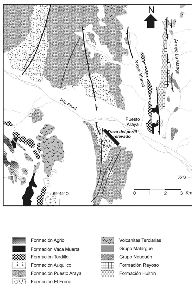
Figura 2. Mapa geológico de la región estudiada, tomado de Gulisano y Gutiérrez Pleimling (1994) / geological map of the studied area, based on Gulisano and Gutiérrez Pleimling (1994).
